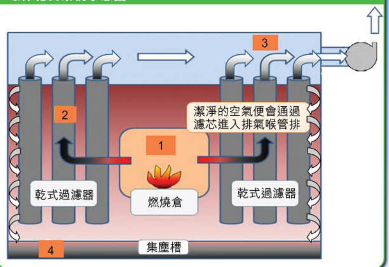
灣仔洪聖廟採用內置乾式煙霧緩減系統的化寶爐。
